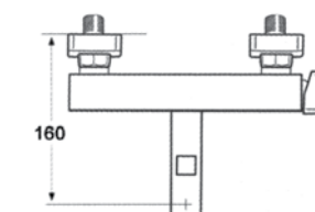
Ref. 121003 Monomando baño ducha Bathtub mixer Acabado cromo Cartucho 35 mm
